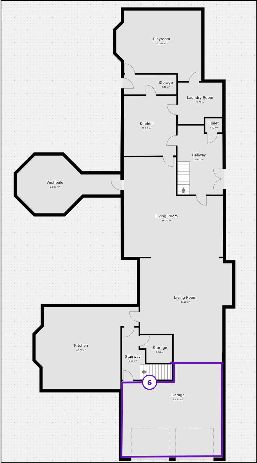
Legende van plan 1.2: WONING/GARAGE - wanden
