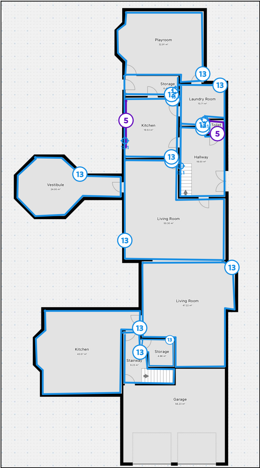
Legende van plan 1.5: GELIJKVLOERS - WONING - Muurpleister.
